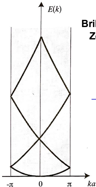
Free Electrons
